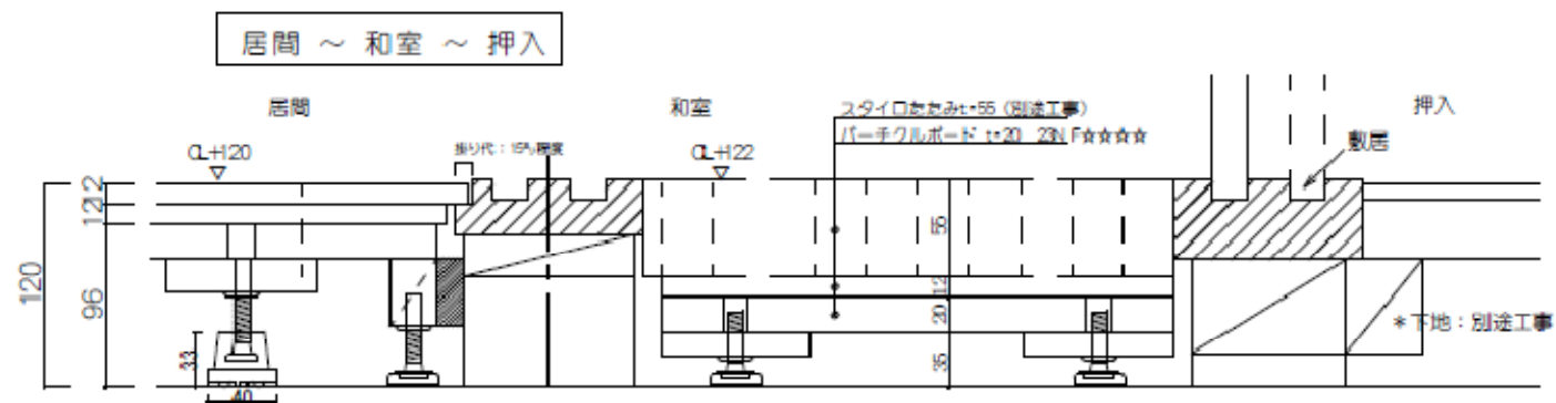
公営住宅 CAD図
