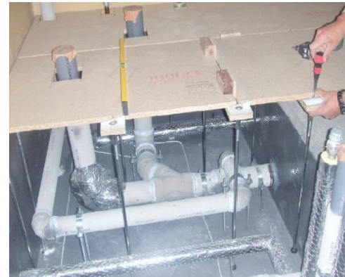
[ 医療センター配管・配線用：ピット部 ]
