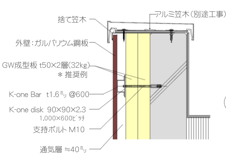
【パラペット部分 断面詳細図】
