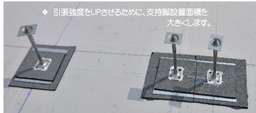
保護材t6 + 保護プレートt2.3 + 保護材t6 (バリキャップ) (ZAM鋼) (バリキャップ)
