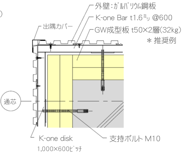
【出隅取合 平面詳細図】
