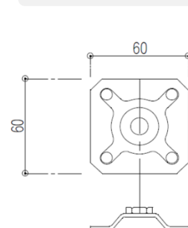
e) PDP ベースプレート
