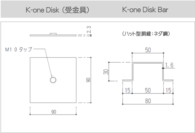
【構成部材：断面図】
