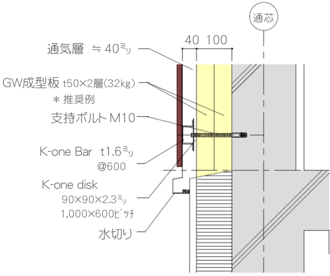
【腰壁部分 断面詳細図】
